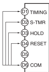
端子台型 (1) (3)
